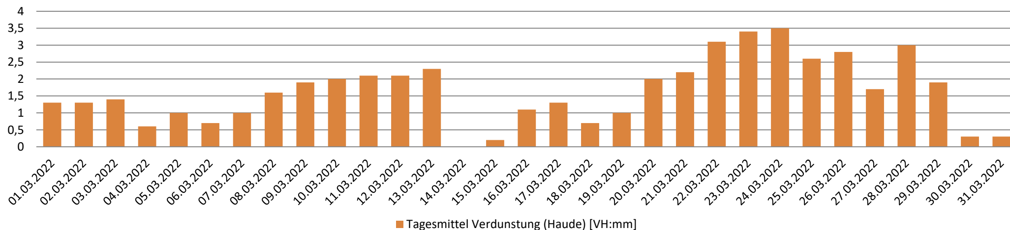
Verdunstung (Haude) [VH:mm]
